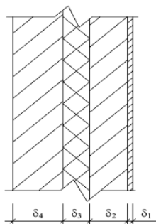
Рисунок – Трехслойная наружная стена
