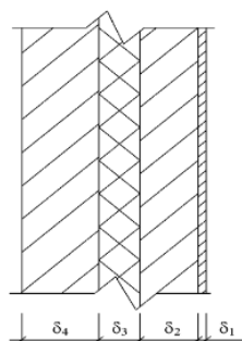
Рисунок – Трехслойная наружная стена
